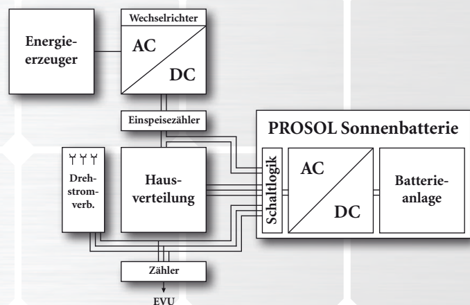
Funktionsweise Sonnenbatterie
