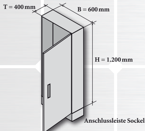
Abmessungen PROSOL Sonnenbatterie 1, 2 und 3
